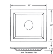
Sump Pans
